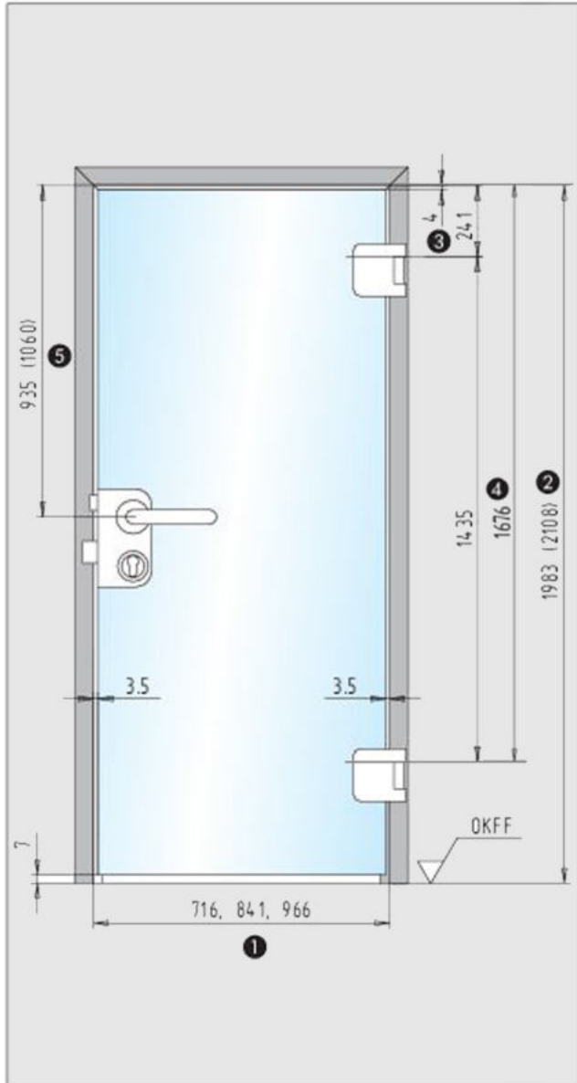
Standard-Glastürblatt mit Zarge
