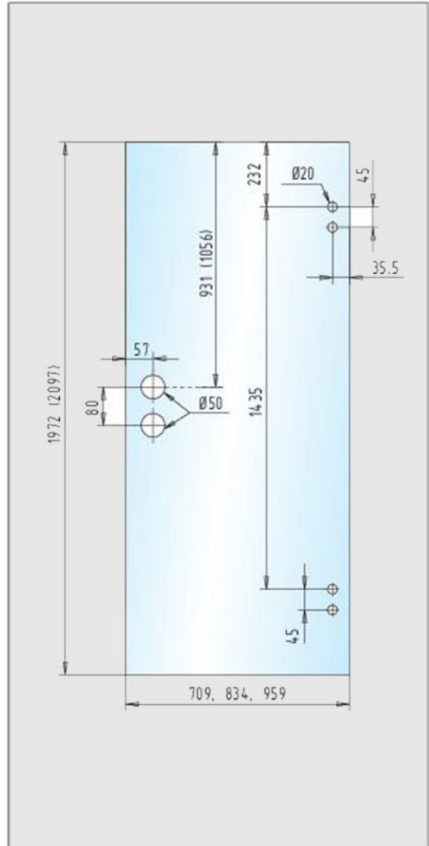
Standard-Türblatt
