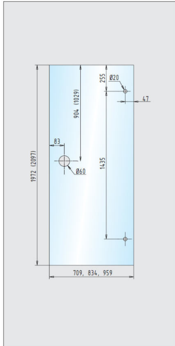
Standard-Türblatt
