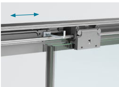
stufenlos einstellbare Dämpferposition infinitely variable damper position
