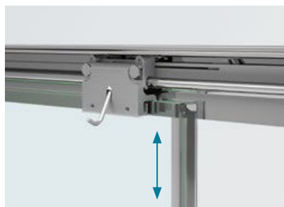
Höhenverstellung height adjustment
