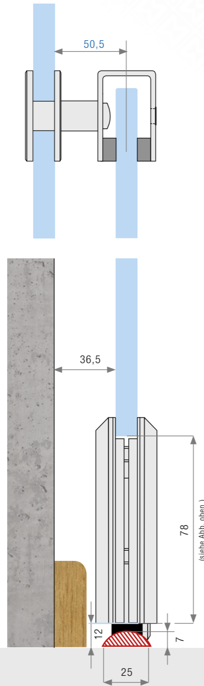
Glastür mit Glasbefestigung und Wandabstandshülse
