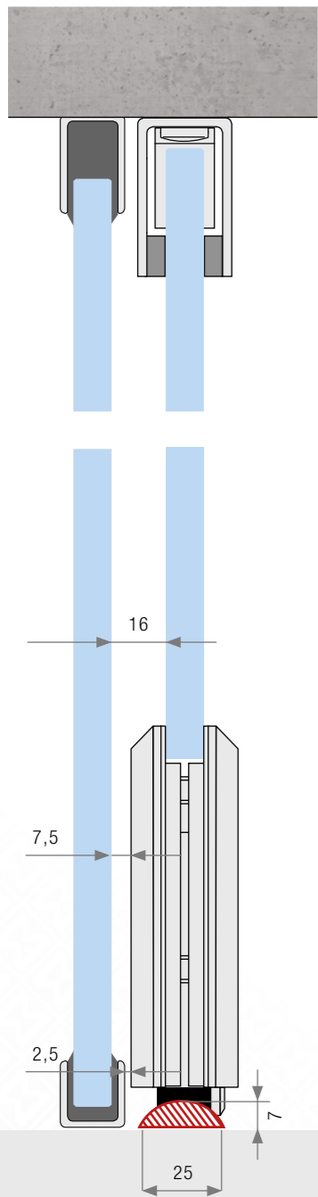
Glastür mit Deckenbefestigung
