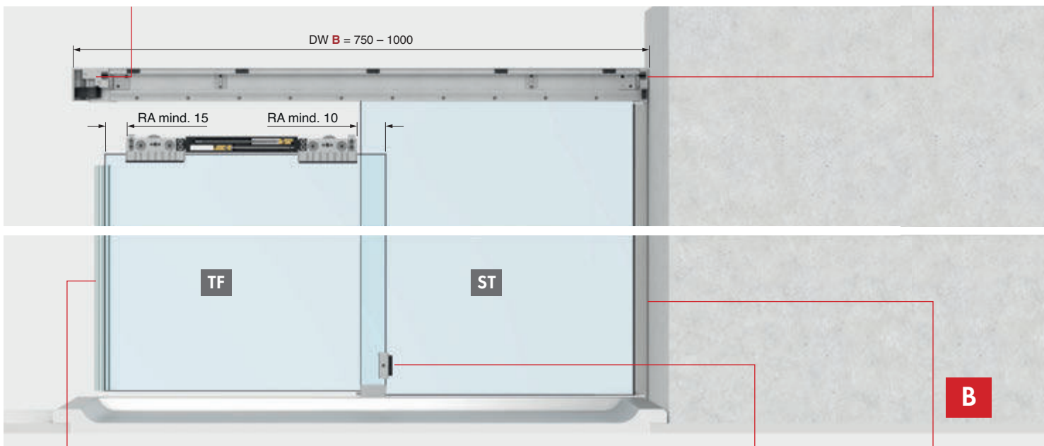
Softstopp doppelseitig (20 kg) softstopp double-sided (20 kg) Art.-Nr.: | art. no.: 8822RAL7016-SSDD-20
