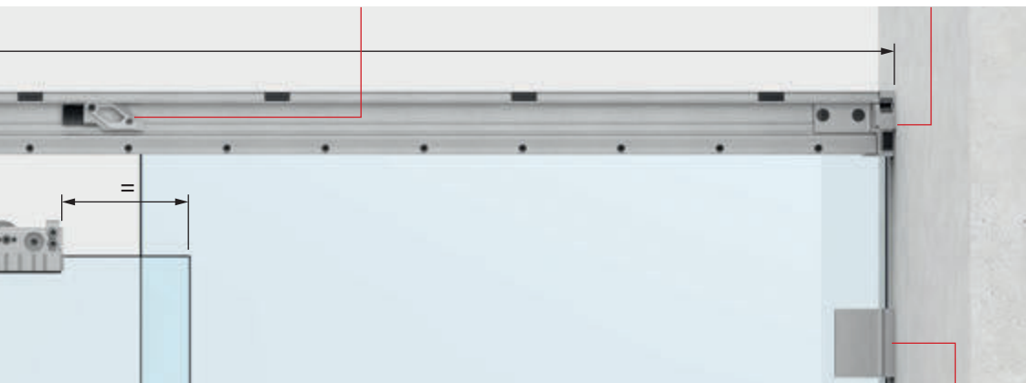
Türanschlag in der Laufschiene door-stop in the guide rail Art.-Nr.: | art no.: 8822ZN_-EA
