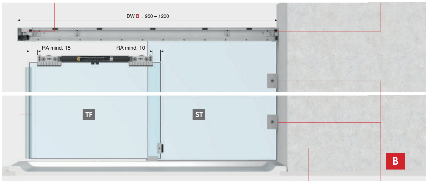
Softstopp doppelseitig (32 kg) softstopp double-sided (32 kg) Art.-Nr.: | art. no.: 8822RAL7016-SSDD
